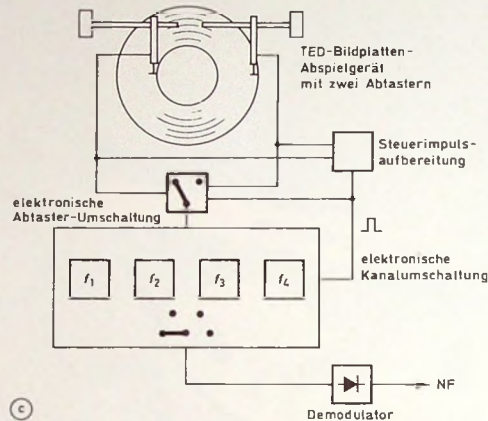
Bild 7. Tonspeicherung mit der TED-Bildplatte (für vier Trägerfrequenzen dargestellt): a) Lage der Filterbereiche, b) Grundschaltung des Verfahrens, c) Schaltung für kontinuierlichen Programmablauf
