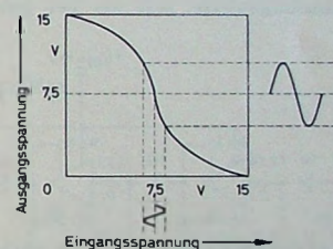
Bild 3. Prinzipieller Verlauf der Übertragungskennlinie einer COS/MOS-Verstärkerstufe
