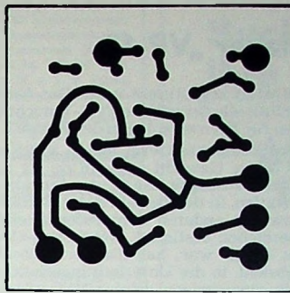
Bild 3. Printplatte des Vorverstär- kers (Maßstab 1 : 1)
