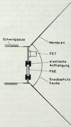
Bild 2. Anordnung der Printplatte mit dem Beschleunigungswandler und dem Feldeffekttransistor-Impedanzwandler im Membranhals des Tiefton-Lautsprechers
