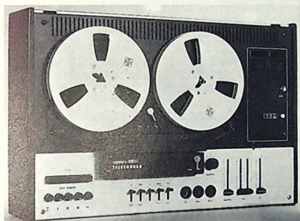
Bild 1. Hi-Fi-Tonbandgerät „magnetophon 3000 hifi“ (tapedeck)
