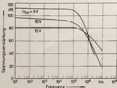
Bild 8. Frequenzgang des dreistufigen COS/MOS-Verstärkers nach Bild 7 bei verschiedenen Betriebsspannungen
