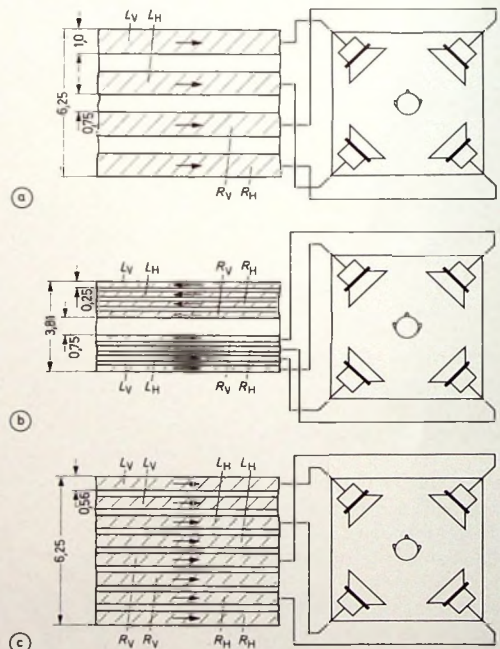
Bild 1. Aufzeichnung der vier Quadro-Kanäle bei den verschiedenen Bandspeichertypen; a) \frac{1}{4} "-Band, b) Compact-Cassette, c) 8-Spur-Kassette
