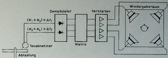
Bild 4. Prinzip der CD-4-Wiedergabeeinrichtung
