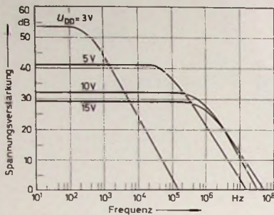
Bild 5. Frequenzgang der COS/MOS-Verstärkerstufe nach Bild 2 für verschiedene Betriebsspannungen U_{DD} (mit R_b = 22 \text{ MOhm} und R_i = 50 \text{ Ohm} )
