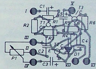
Bild 8. Bestückungsplan des Baßkanals
