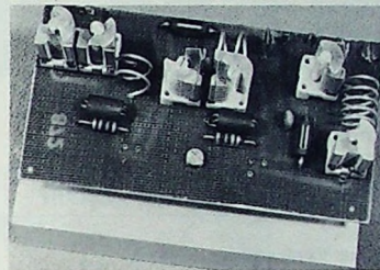
Bild 2. Sender-Endstufen-Baustein „FA 145“ für das 2-m-Band (Conrad)
